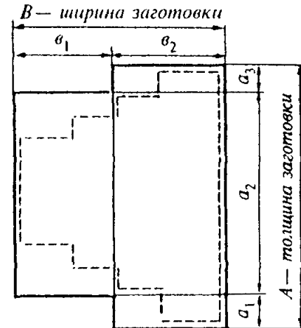
Рисунок 2 - Примеры сечений двух- и трехслойных брусковых заготовок для оконных блоков по ГОСТ 24700
