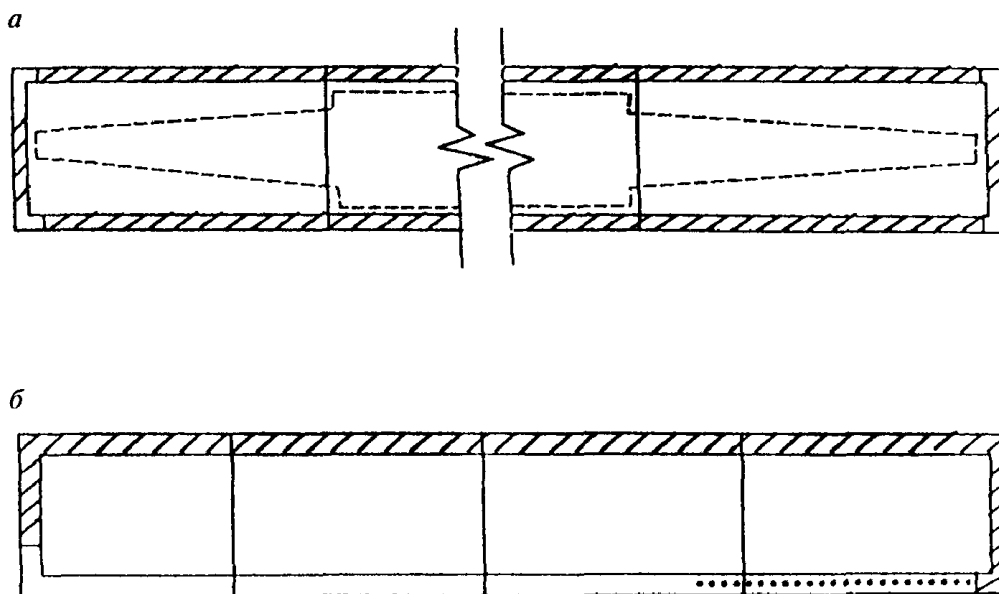
Рисунок 7 - Примеры определения видов поверхностей заготовок и деталей для оконных блоков по ГОСТ 24700
